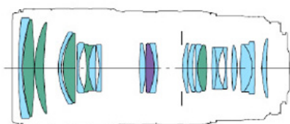
● Lente Fluorita ● Lente UD
