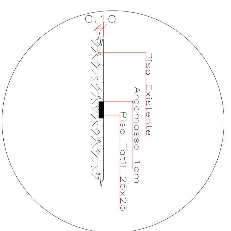
Detalhe 02
